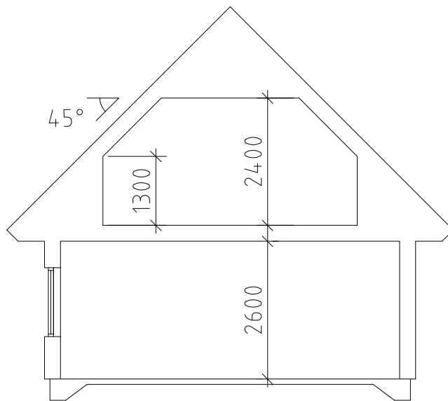
SEKTION A-A
